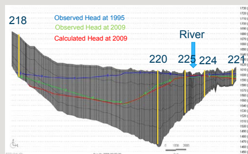
مدل آب های زیرزمینی: FEFLOW برش های مقطعی در زیر حوضه نجف آباد
