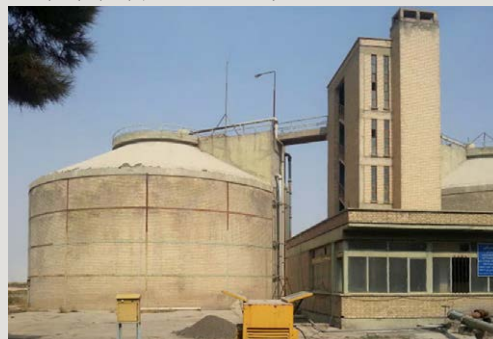
تصفیه خانه فاضلاب شمال اصفهان، دجیستر فاز ۱
